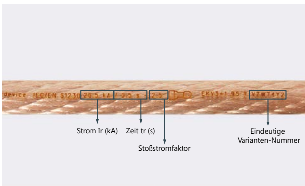
Notwendige Kennzeichnung der EuK-Vorrichtung (siehe Laserung anbei)
